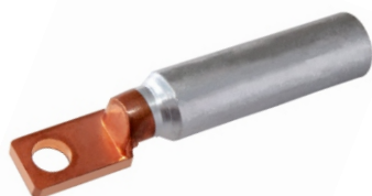
Conector de pala angosta para breaker totalizador
